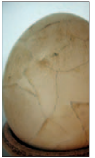
Σταυρολίτης, Ρωσία. 35-40 εκατομμυρίων ετών. Δεξιά αβγά δεινοσαύρου.
